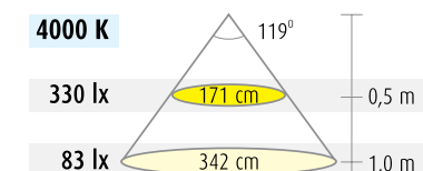
VALONJAKOKÄYRÄ
